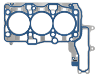
192.650 # 11 12 8 594 563 1,45 mm | 3-layer
